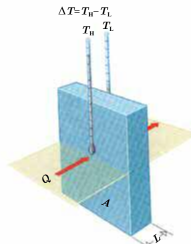
شکل ۴-۳ تیغه‌ای به ضخامت L و مقطع A بین دو منبع با دماهای T_L و T_H قرار گرفته است.
