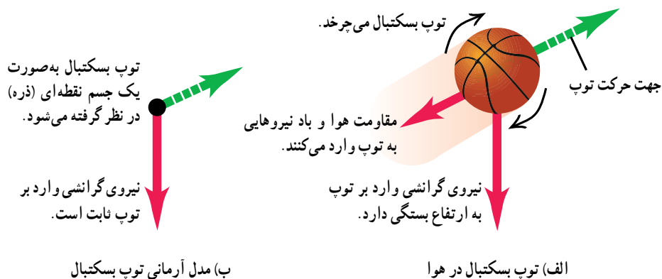
شکل ۳-۱ استفاده از یک مدل آرمانی برای ساده‌سازی تحلیل حرکت یک توپ بسکتبال در هوا
