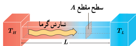
شکل ۴-۳۰ میله‌ای به طول L و مقطع A بین دو منبع بادماهای T_L و T_H قرار گرفته است.
