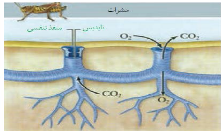
شکل ۲۱- تنفس نایدیسی
